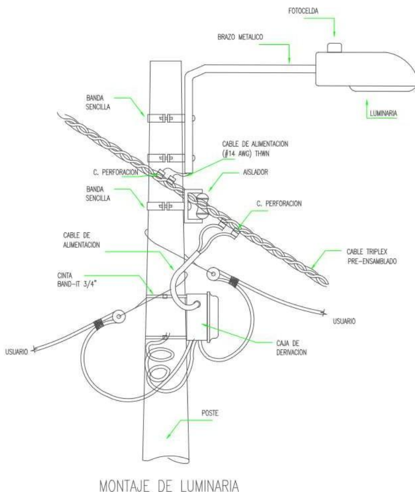
Fig. 1. Esquema montaje de Luminarias
